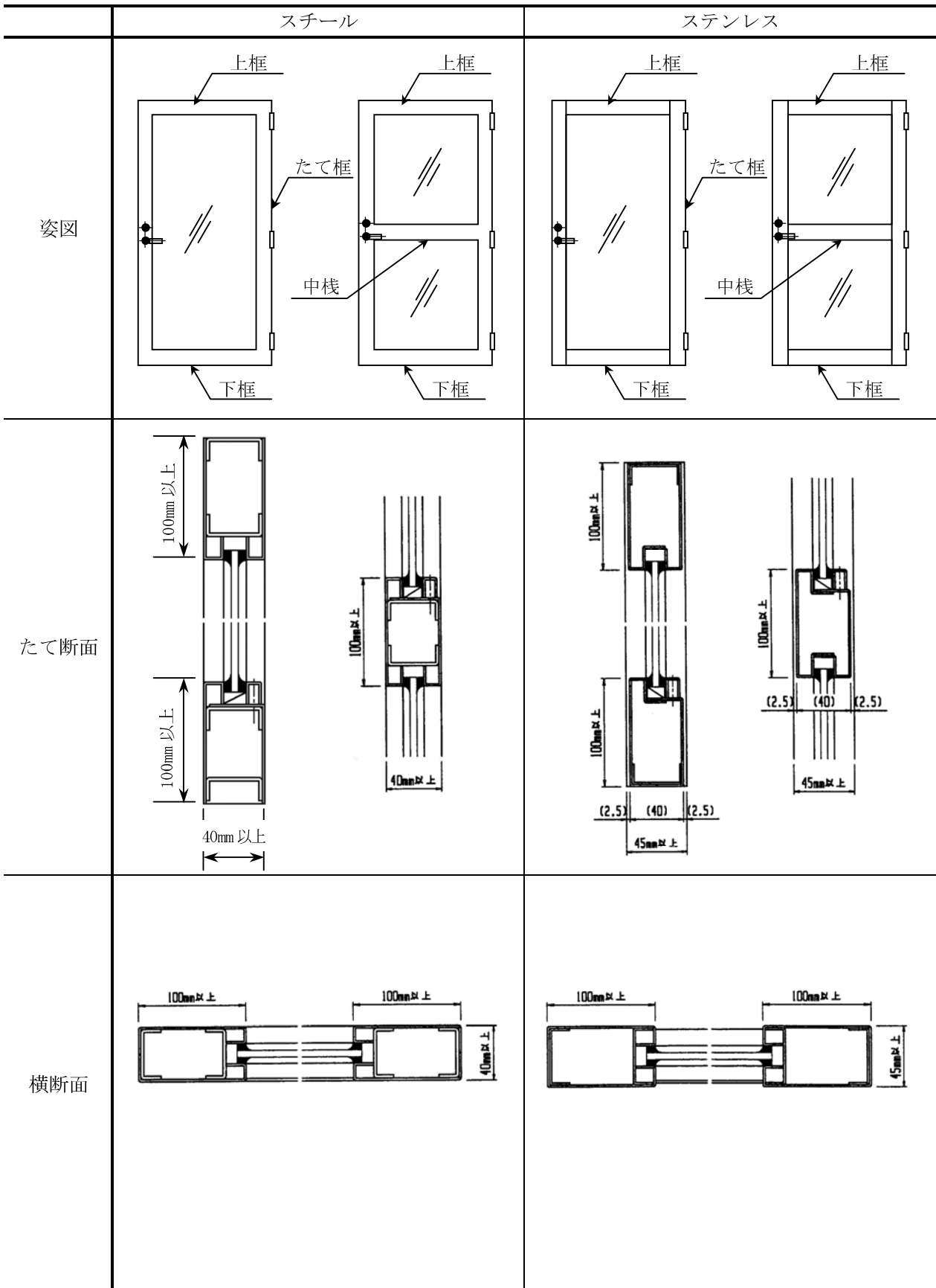
図3 形状及び見付・見込寸法(2)
