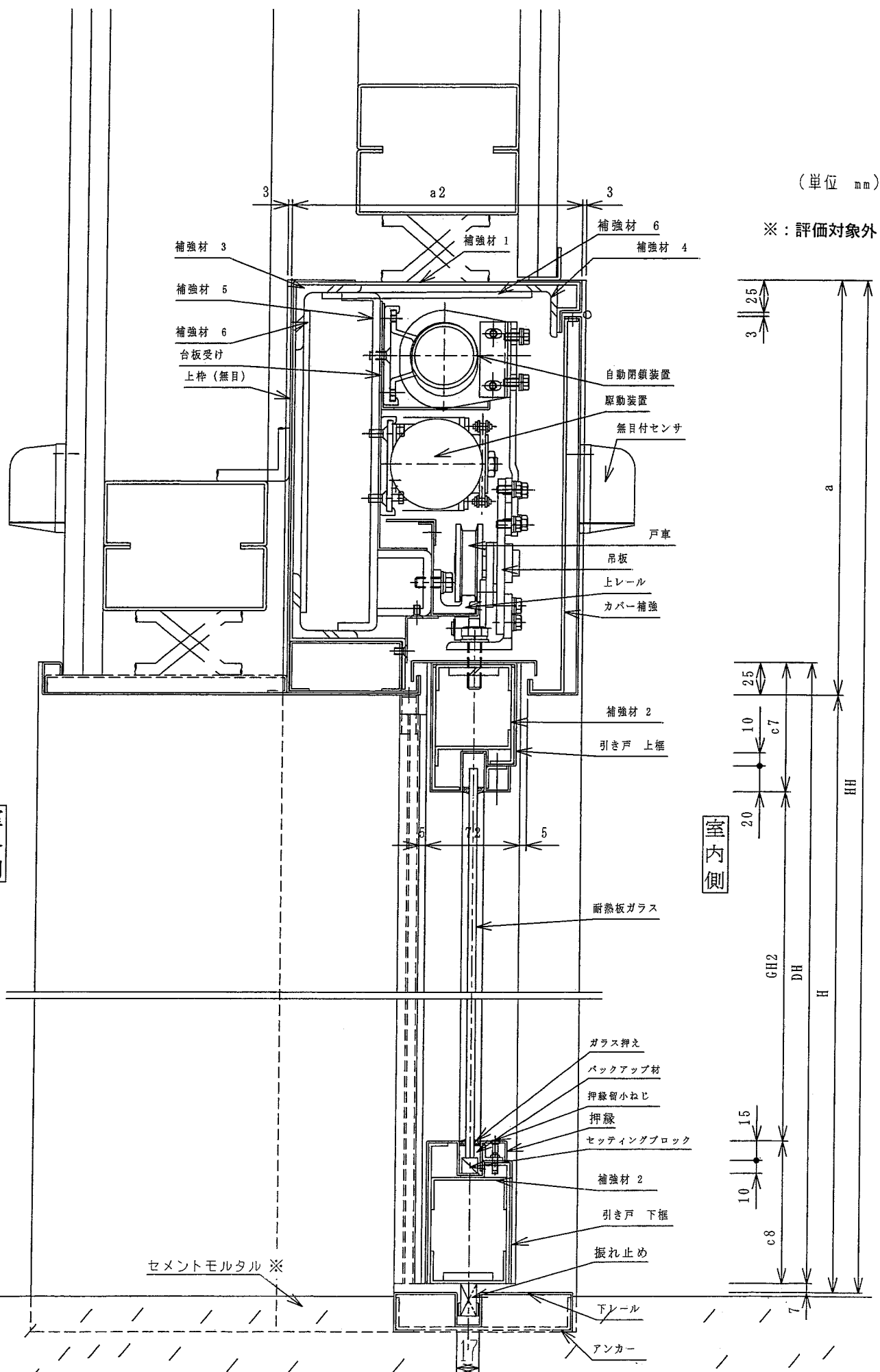
鉛直断面図 (乾式工法、開き戸機構無し、片袖ボード施工仕様)
