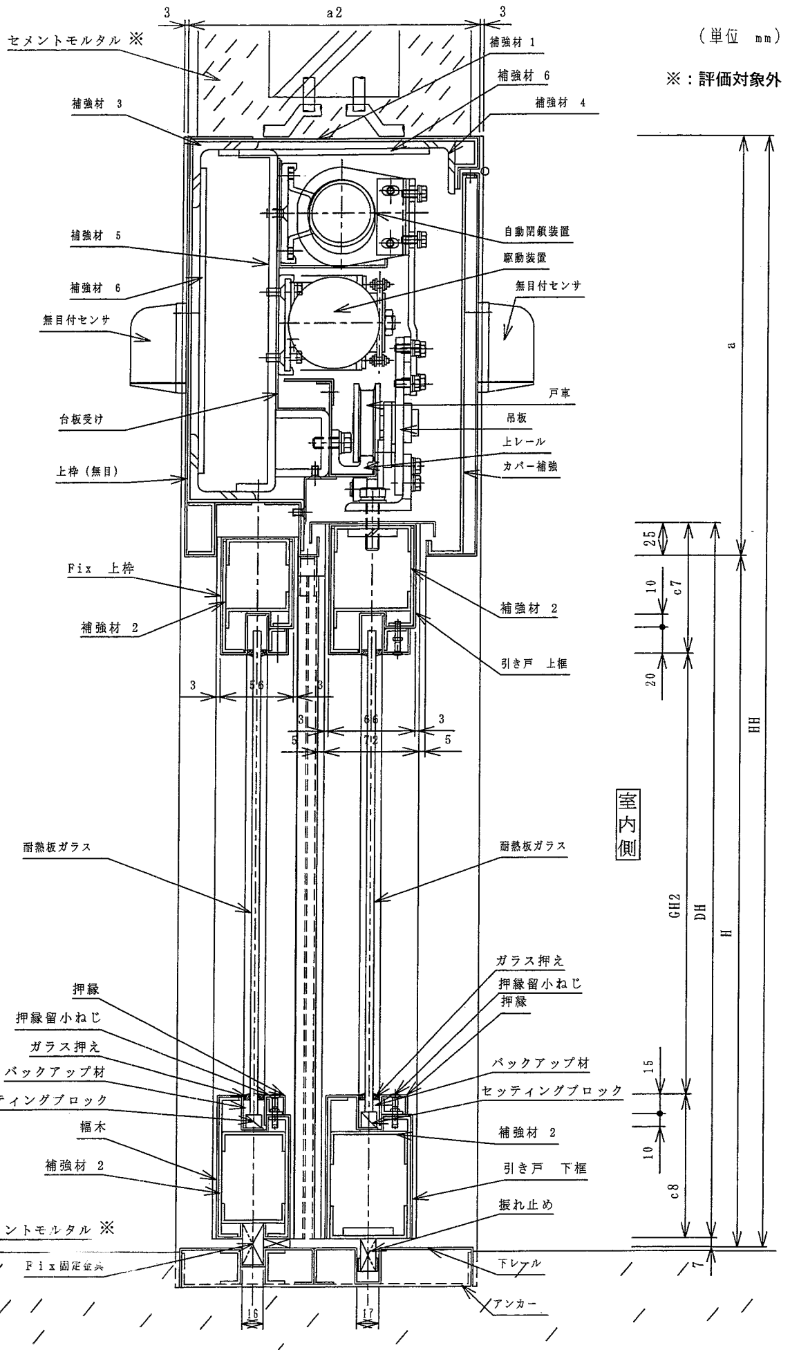
鉛直断面図 (湿式工法、開き戸機構無し、片袖ガラス施工仕様)
