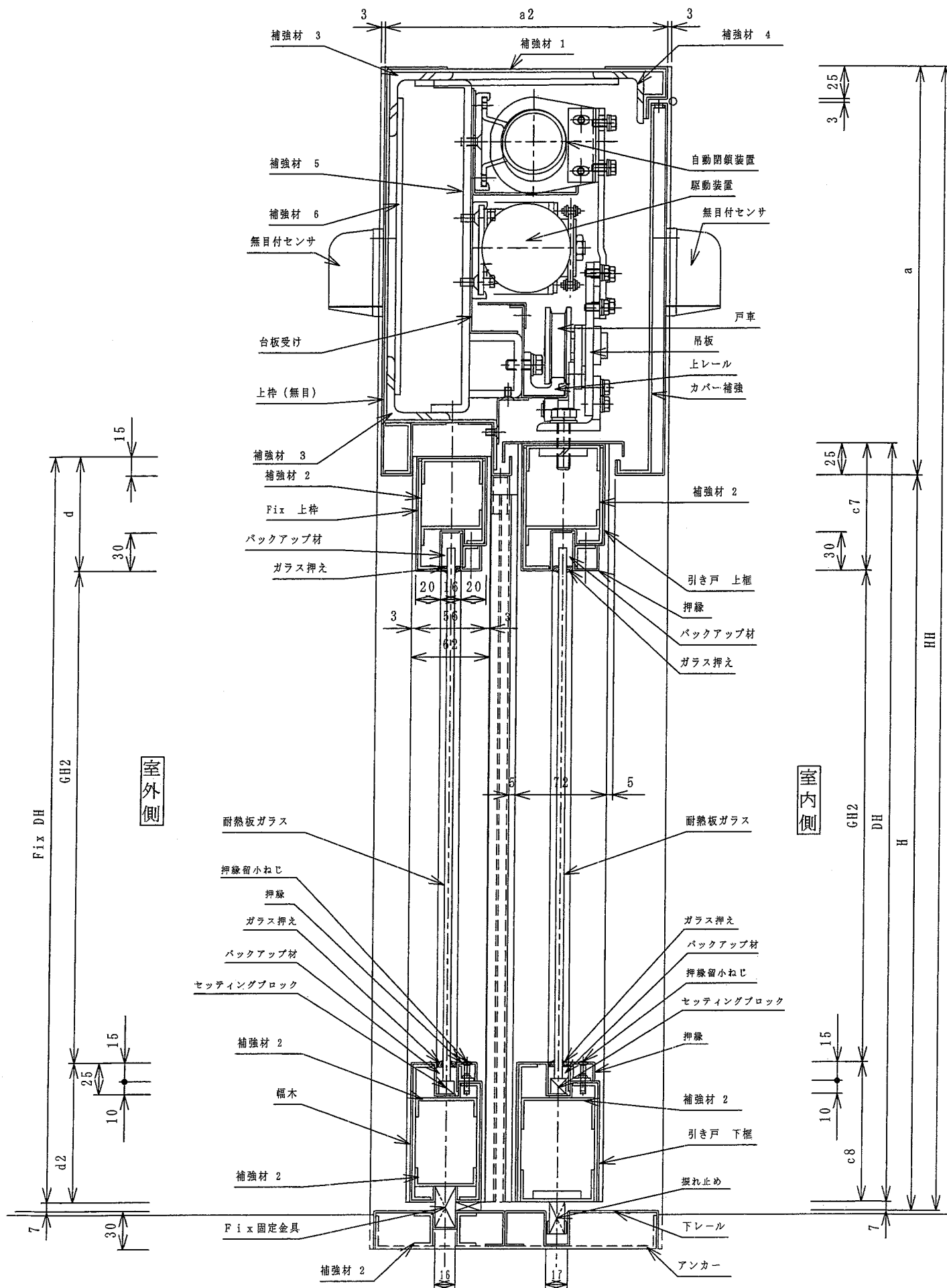
鉛直断面図（開き戸機構無し） 図7構造説明図
