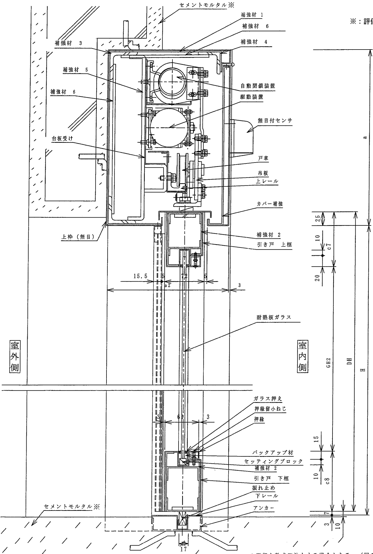
鉛直断面図 (湿式工法、開き戸機構無し、片袖壁施工仕様)
