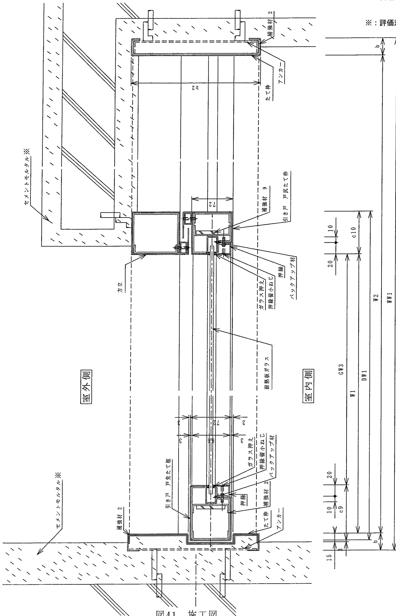
図41 施工図
