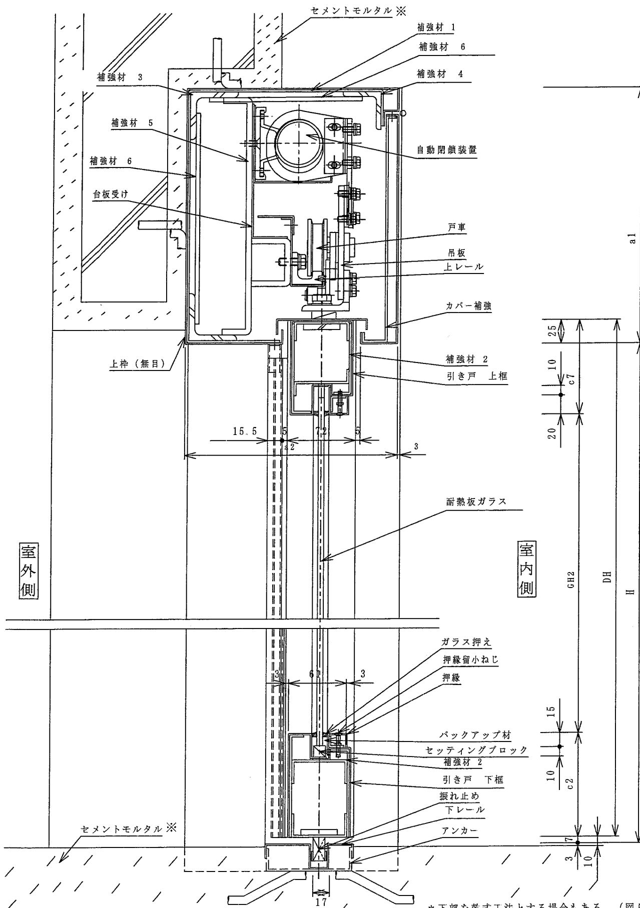
鉛直断面図 (湿式工法、開き戸機構無し、片袖壁施工仕様)
