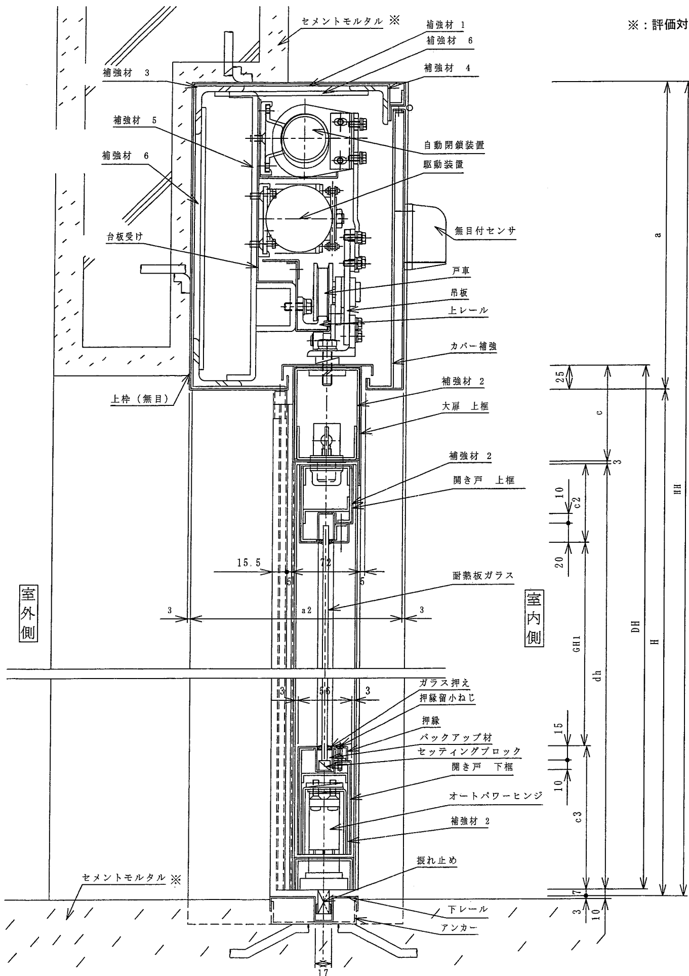
鉛直断面図 (湿式工法、開き戸機構付、片袖壁施工仕様)
