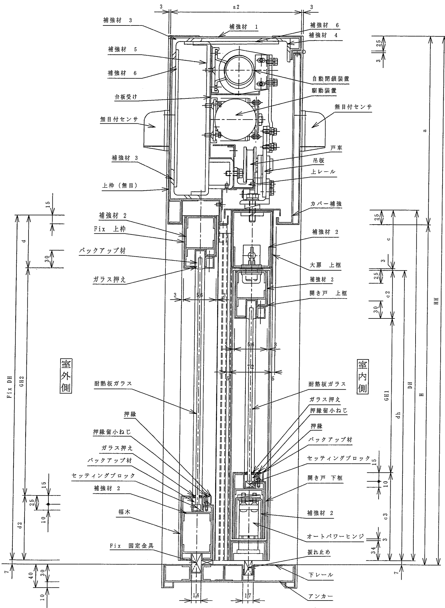
鉛直断面図 (開き戸機構付)
