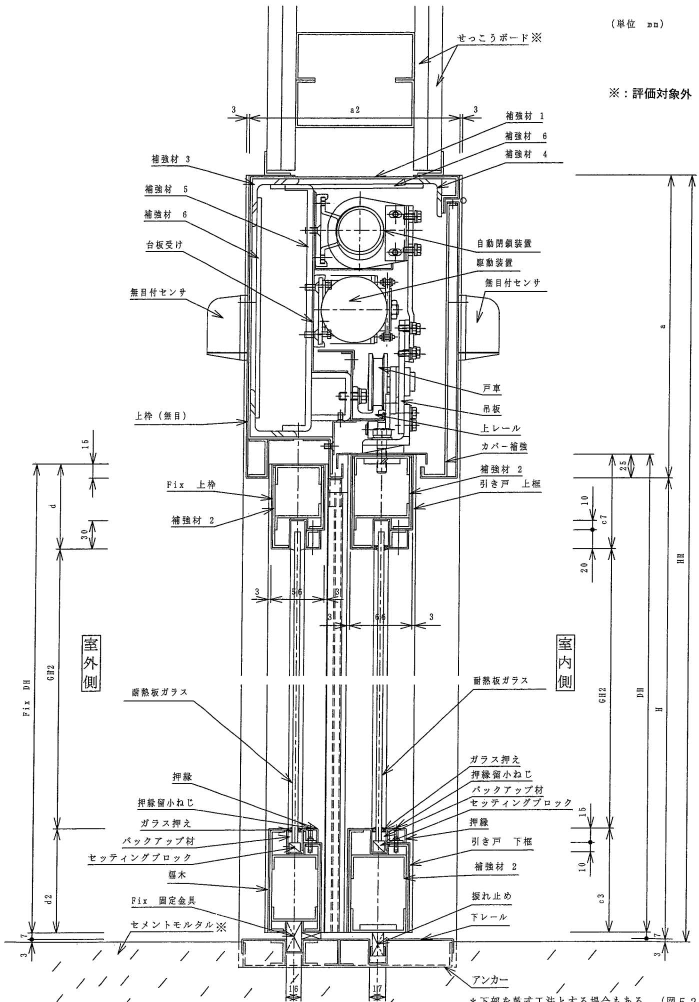
鉛直断面図 (乾式工法、開き戸機構無し、片袖ガラス施工仕様)
