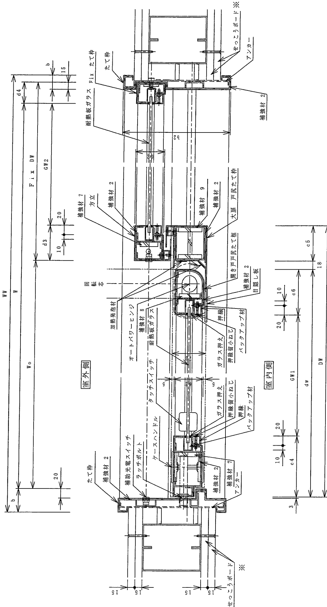
図27 施工図
