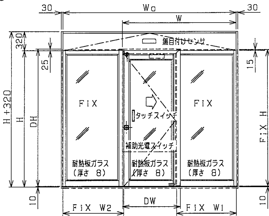
立面图
