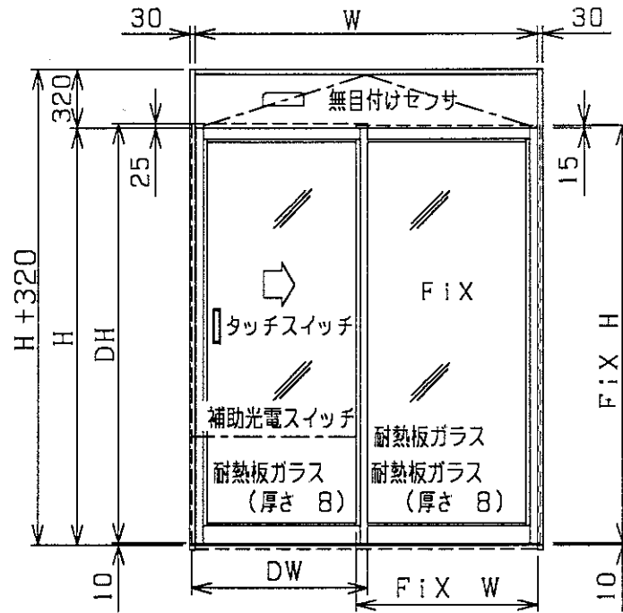
立面图
