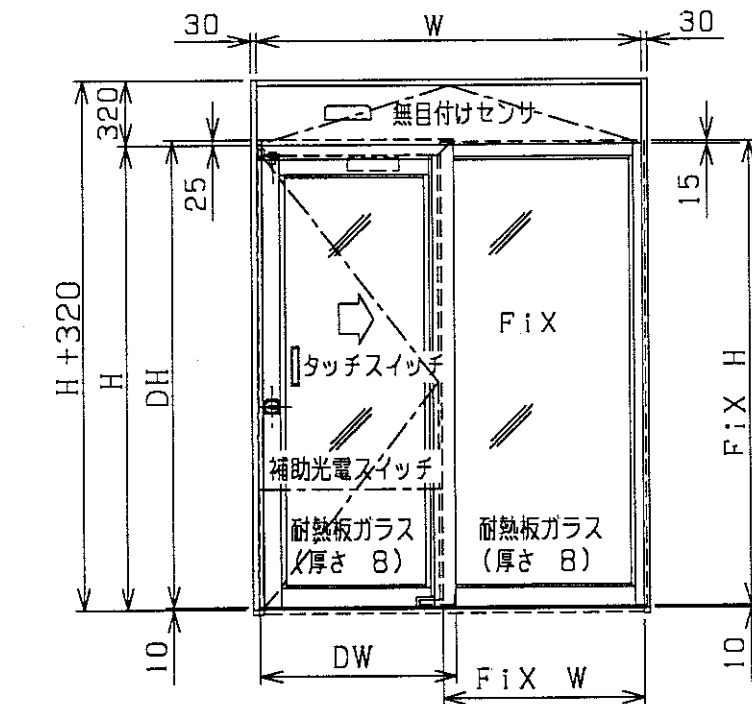
立面図
