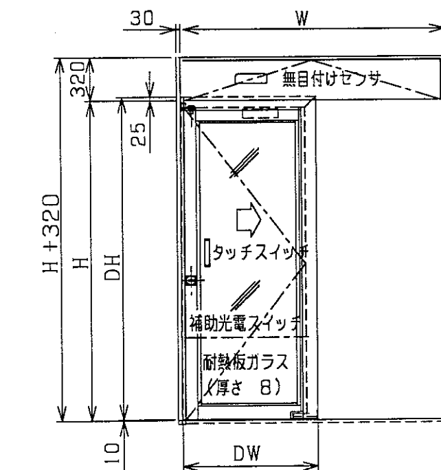
立面図
