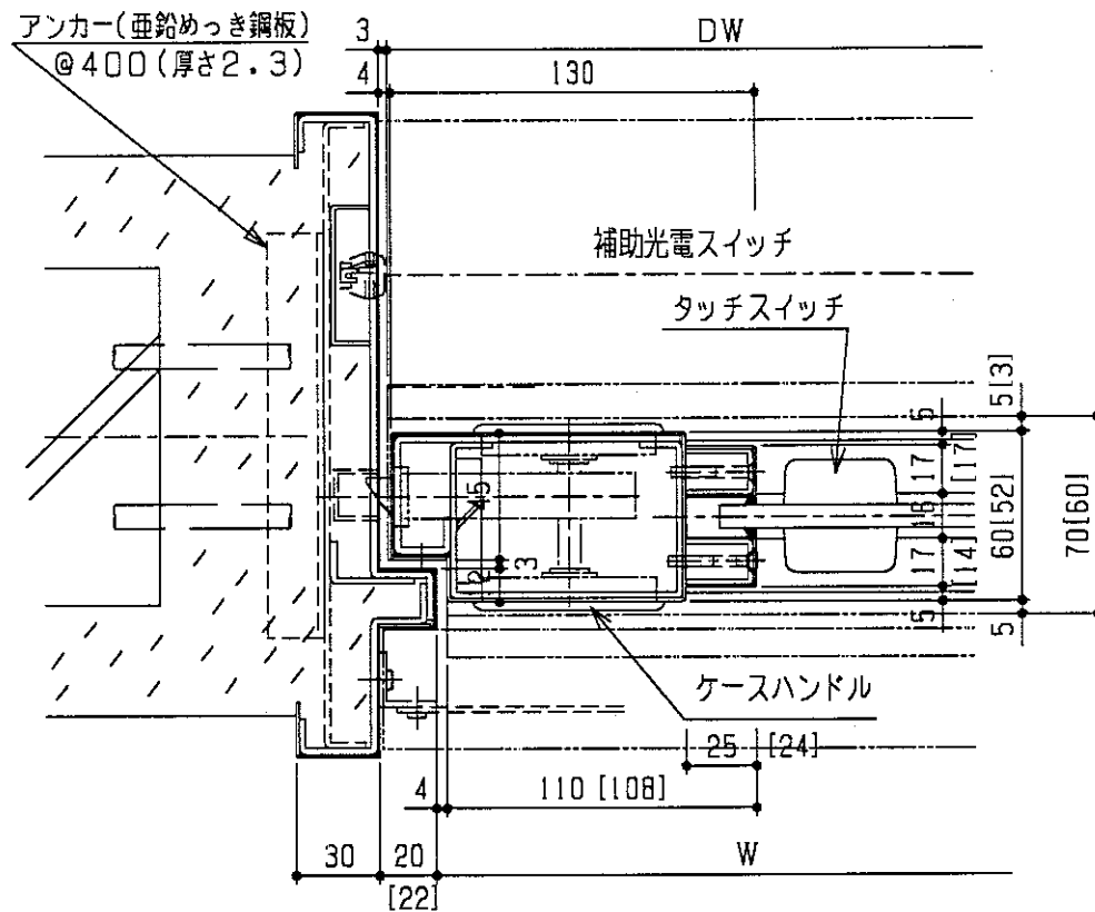
⑭ 片引き戸 水平断面図(片袖はめ殺し)
