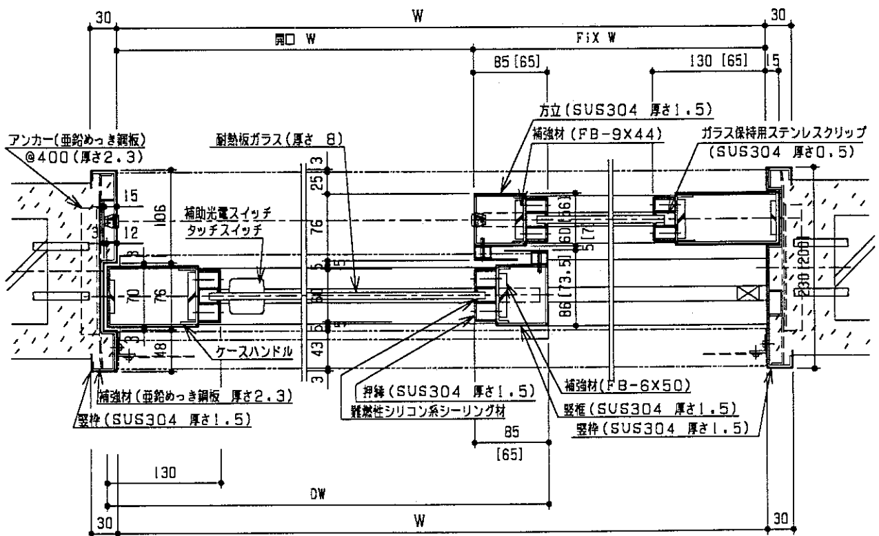
⑭ 片引き戸 水平断面図(片袖はめ殺し)
