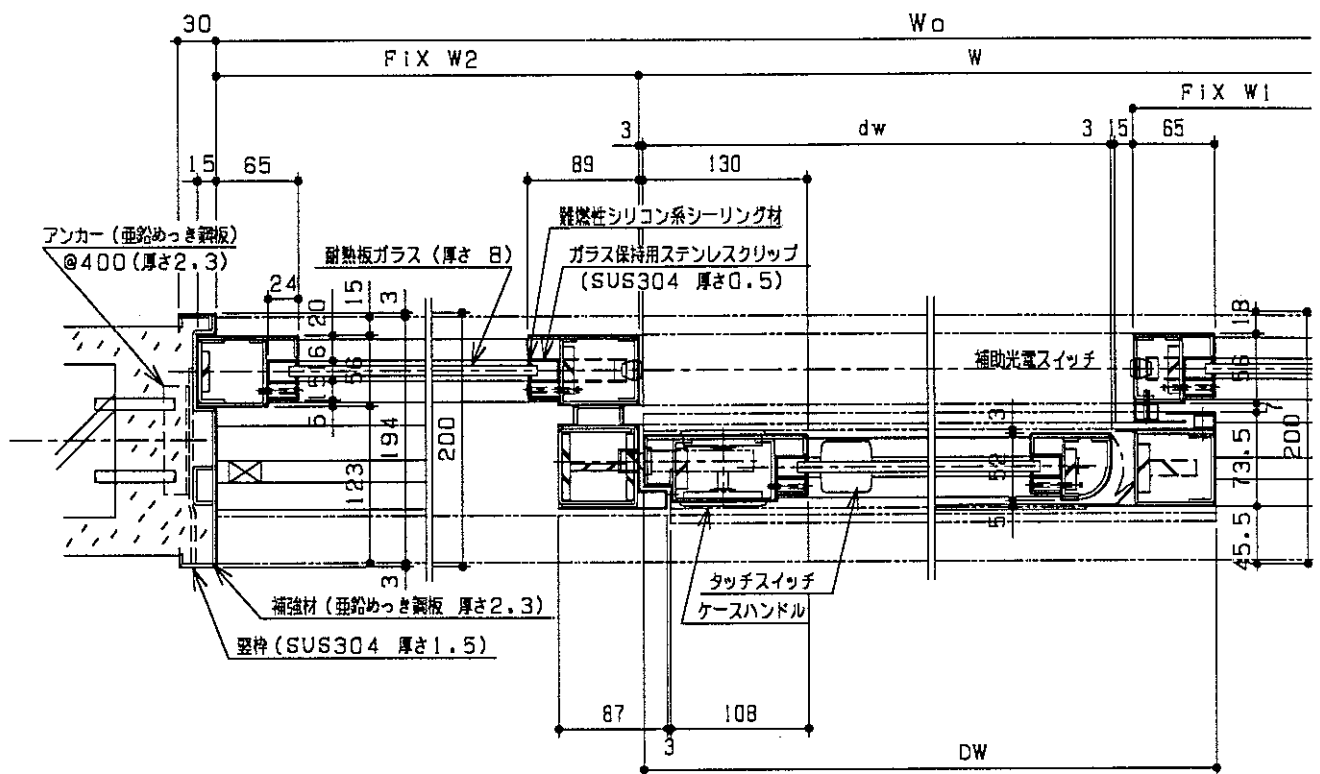
⑬ 片引き戸 (両袖はめ殺し) 水平断面図
